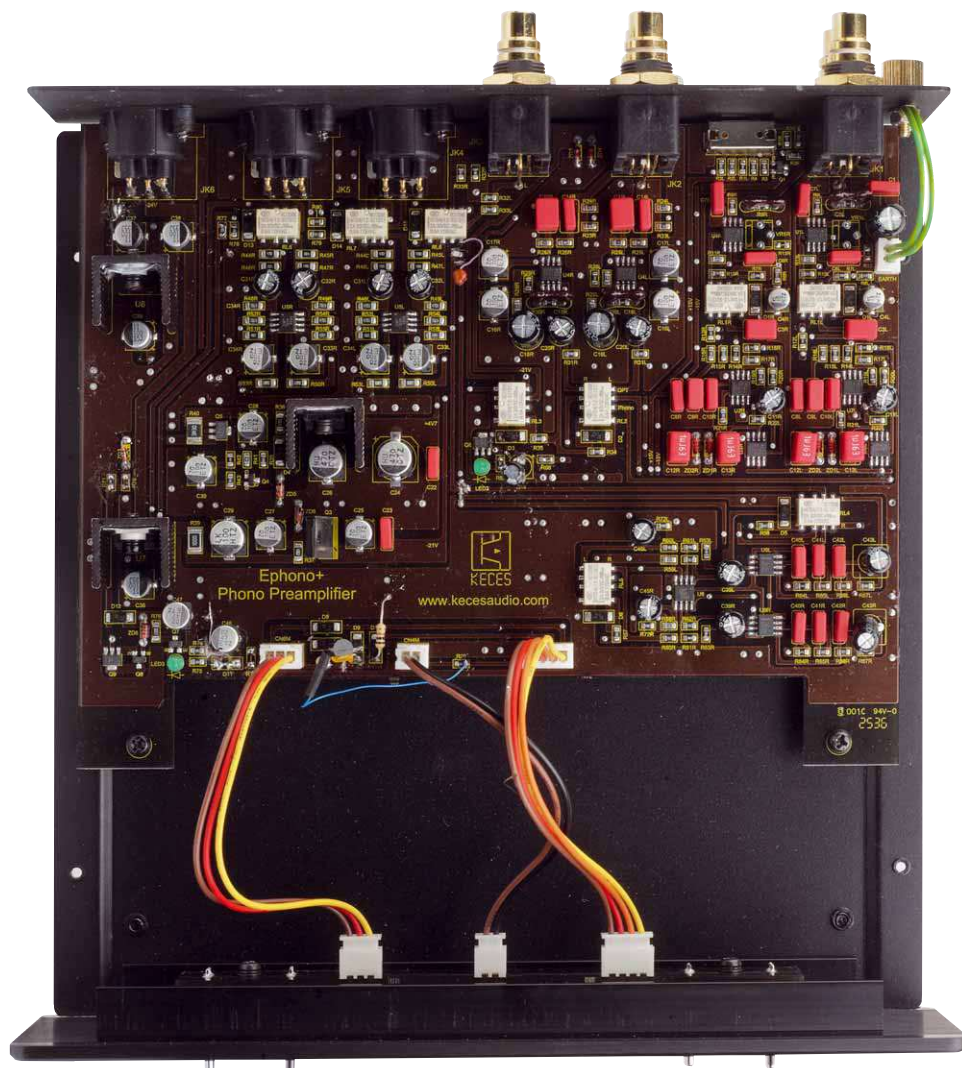
Moderne Technik aus dem Keces-Labor. Viel SMD, viele Regler, am Ende sehr viel Klang
